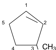
(3-metilciclopenteno)
