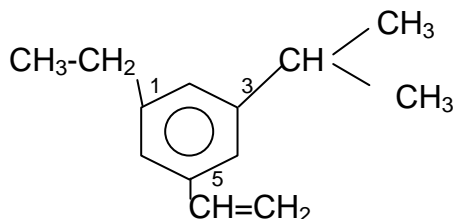
1-etil-3-isopropil-5-vinilbenceno
