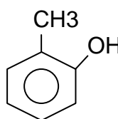
o-metilfenol
