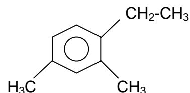
1-etil-2,4-dimetilbenceno
