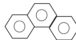
Fenantreno
