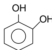
o-dihidroxibenceno o-hidroxifenol
