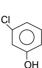
m-clorofenol
