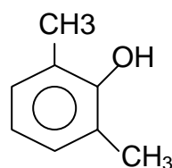
2,6-dimetilfenol
