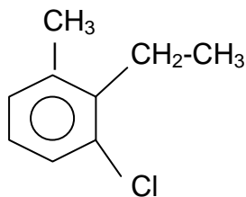
1-cloro-2-etil-3-metilbenceno
